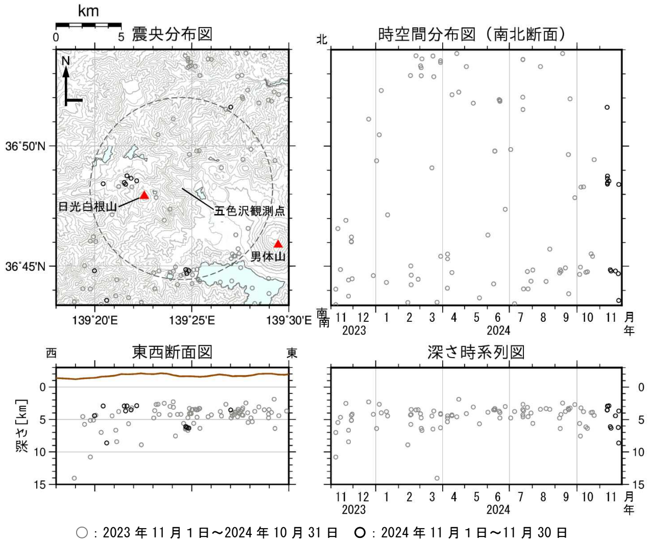
図3 日光白根山 広域地震観測網による山体周辺の地震活動 (2023 年 11 月 1 日～2024 年 11 月 30 日)
