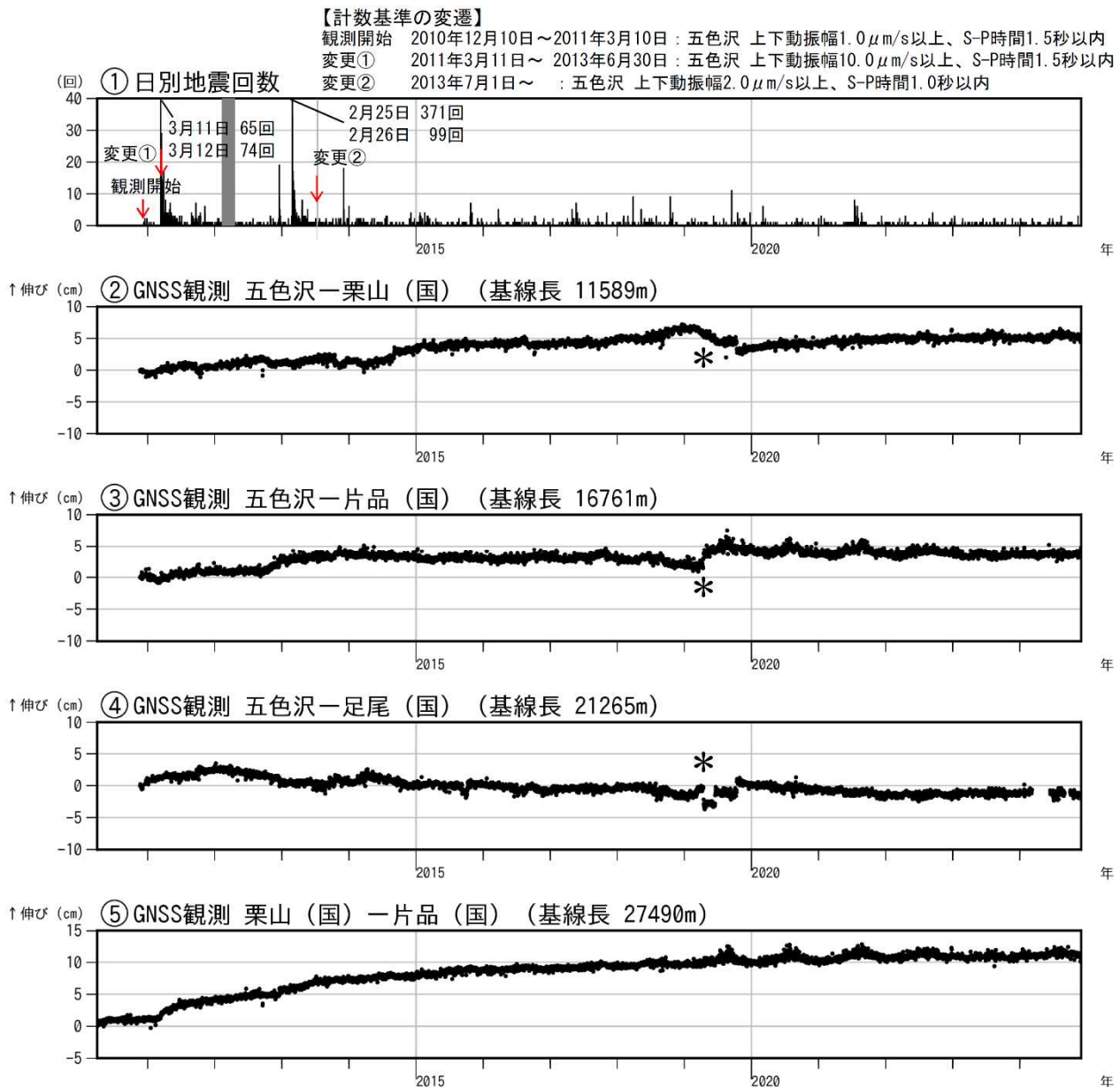
図2 日光白根山 火山活動経過図（2010年4月1日～2024年11月30日）
