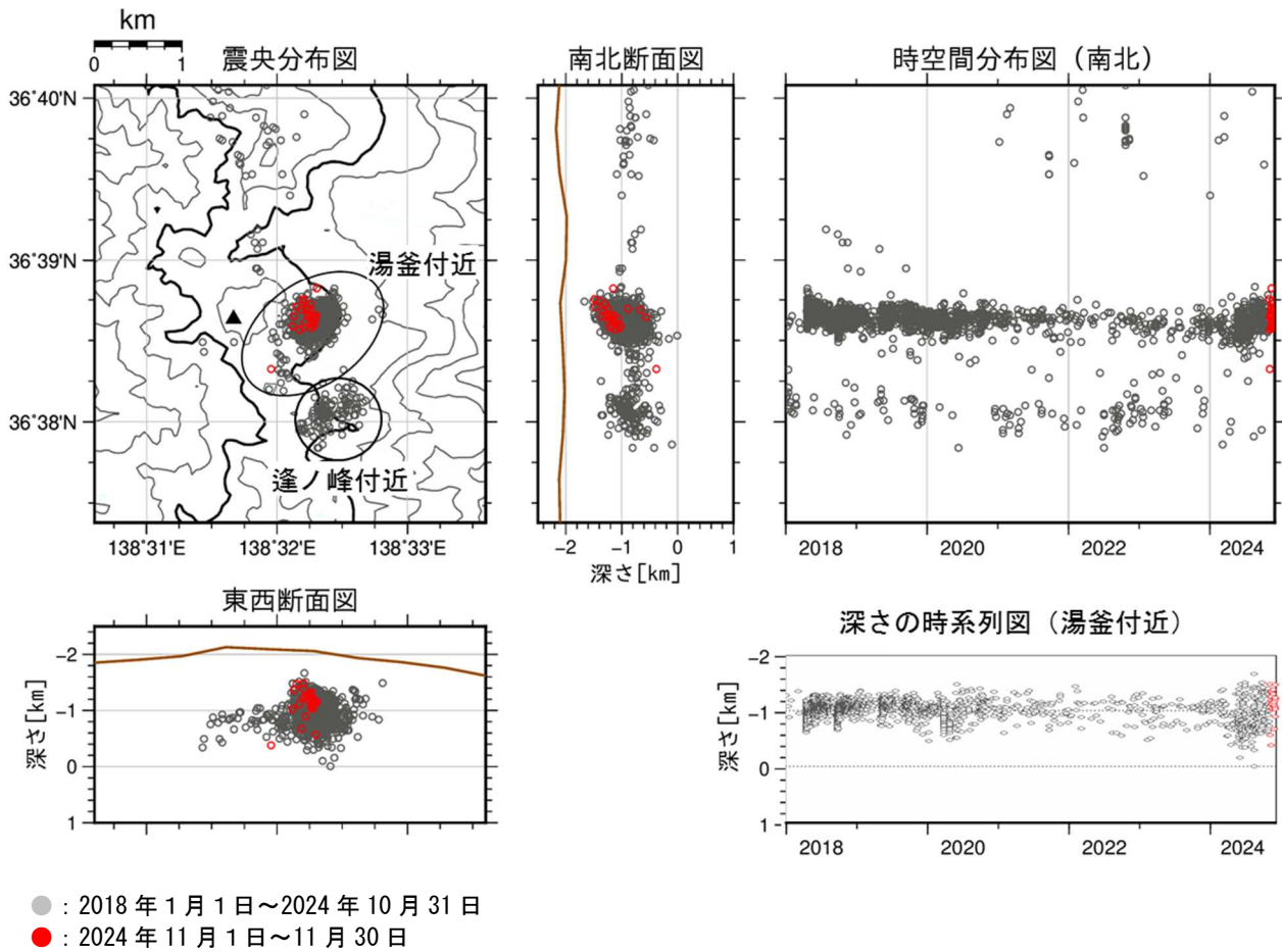
図4 草津白根山 震源分布図（2018 年 1 月 1 日～2024 年 11 月 30 日）
