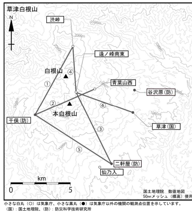
図7 草津白根山 GNSS 観測点配置図
