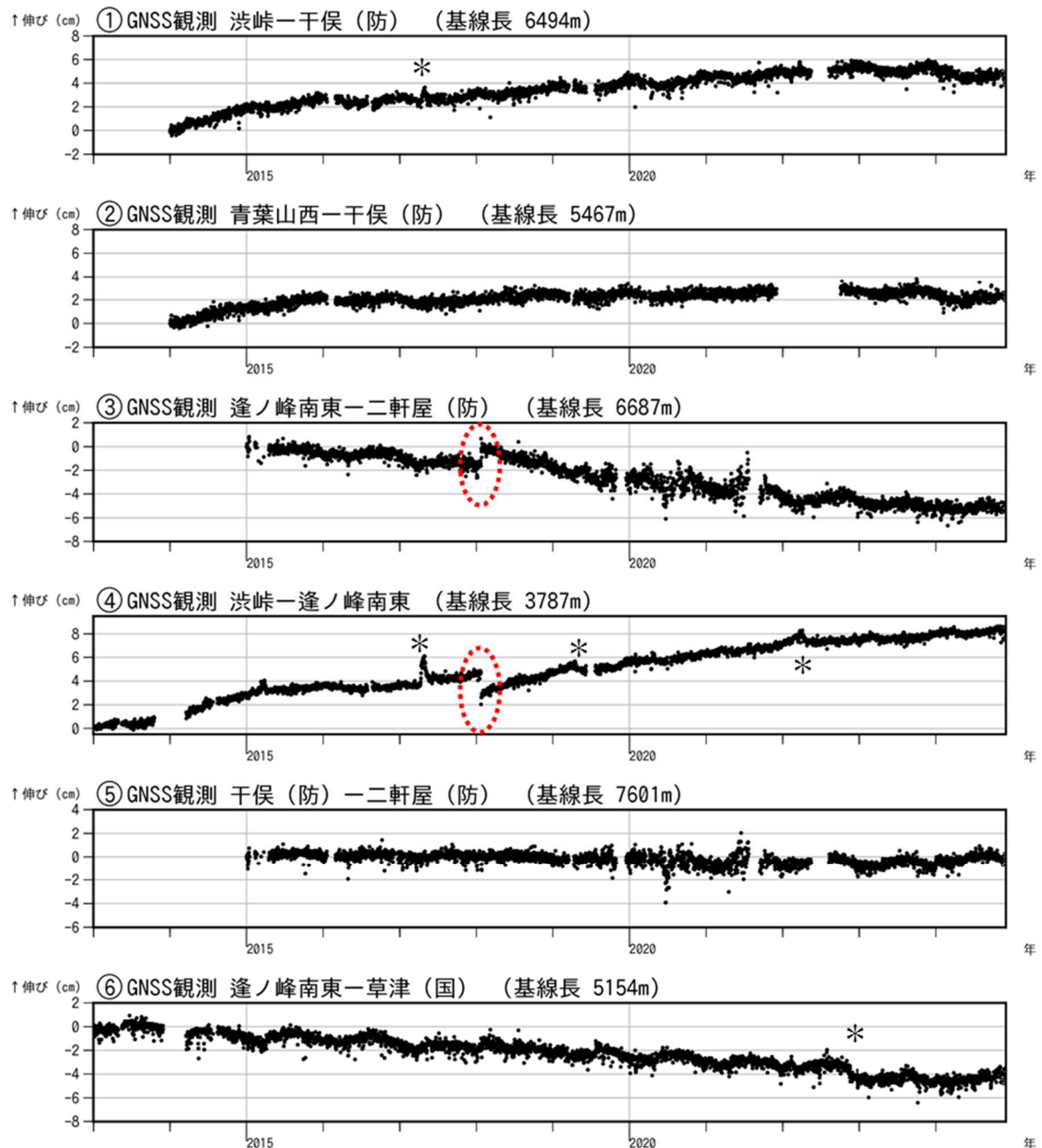
図6 草津白根山 GNSS 連続観測の結果（2013 年 1 月 1 日～2024 年 11 月 30 日）
