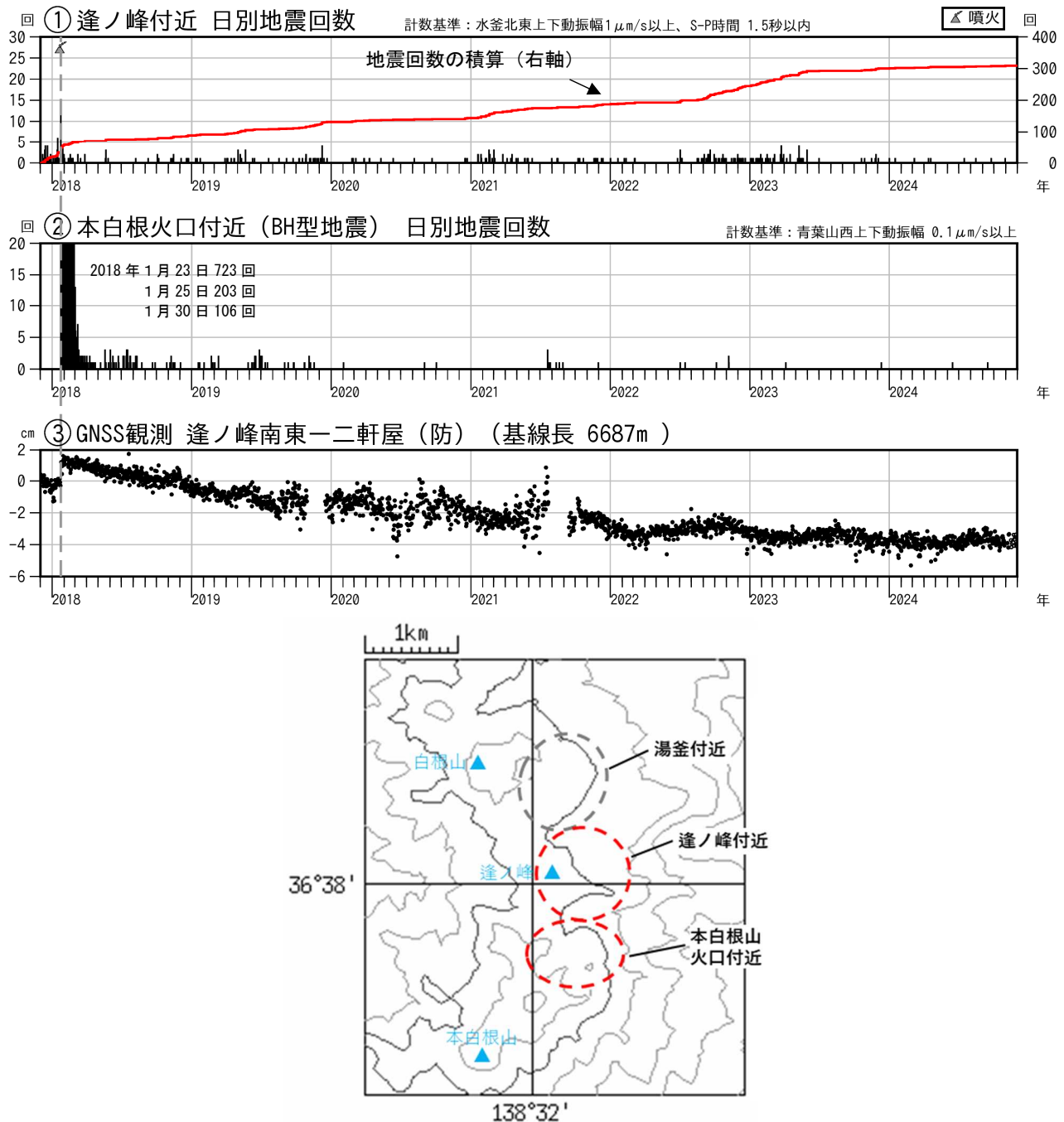
図13 草津白根山（本白根山） 火山活動経過図（2017年12月1日～2024年11月30日）
