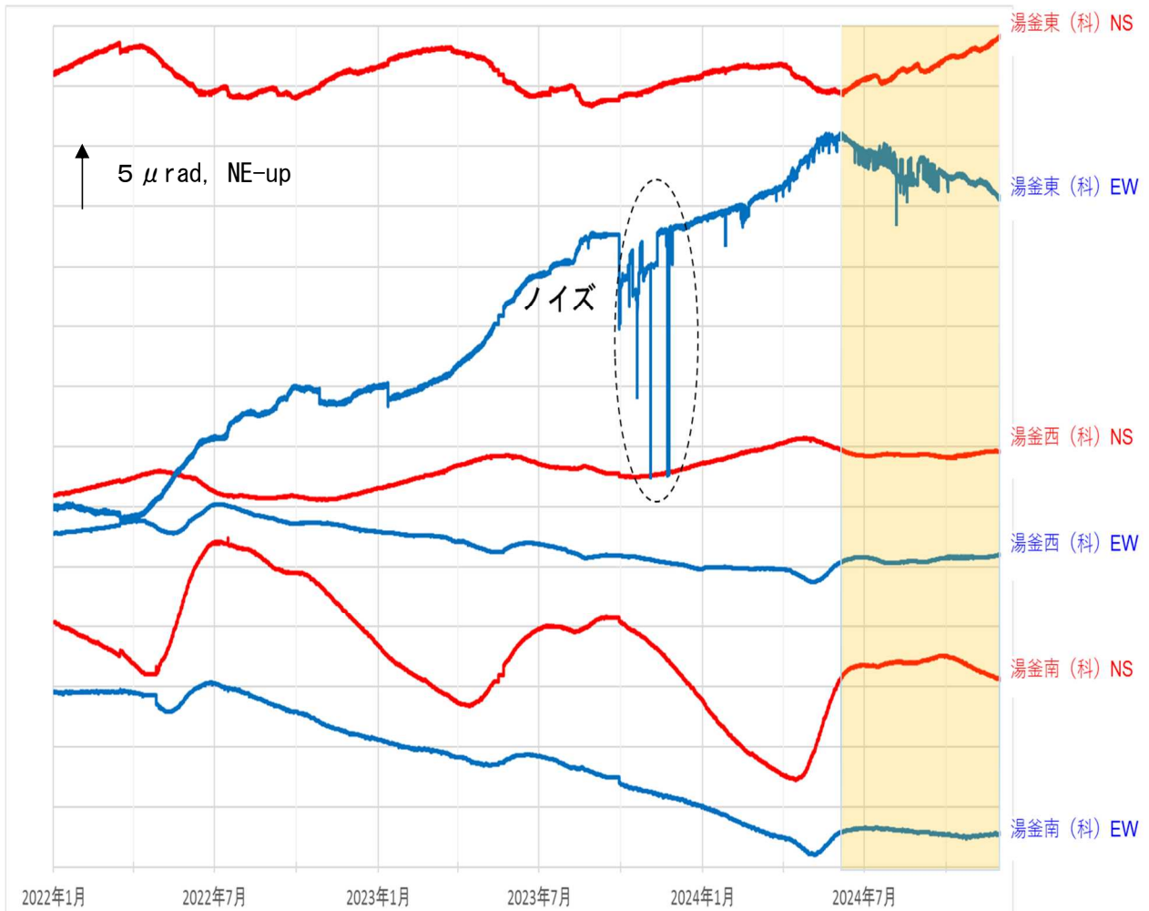
図5 草津白根山（白根山（湯釜付近）） 傾斜変動（2022年1月1日～2024年11月30日）
