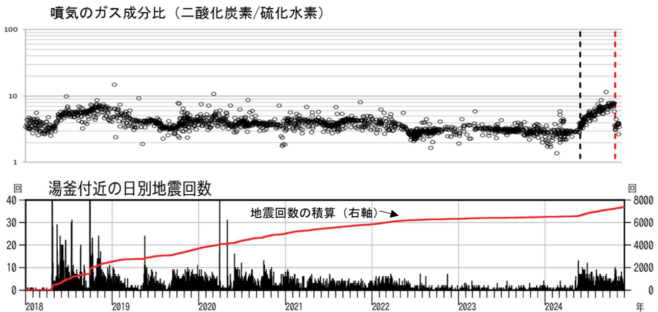
図8 草津白根山（白根山（湯釜付近）） 火山ガス観測結果（2018年1月～2024年11月）
