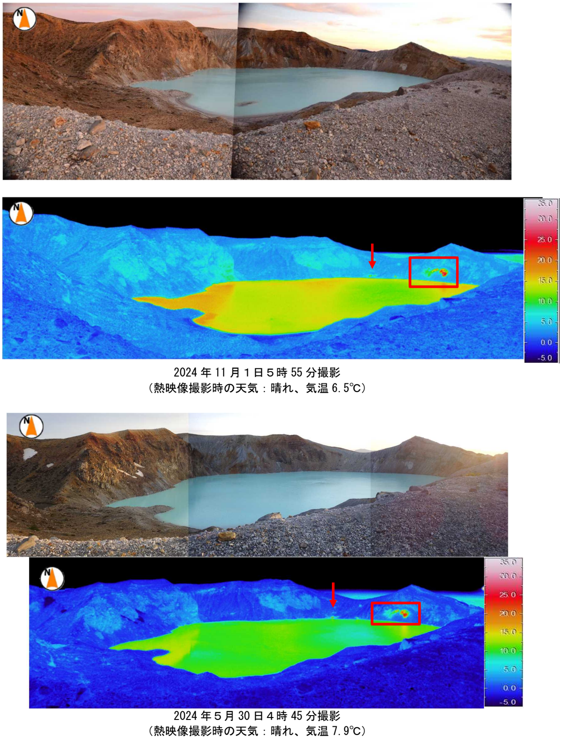
図 2－3 草津白根山（白根山（湯釜付近））湯釜火口内の状況 日射の影響のない早朝に観測された結果を比較しています。
