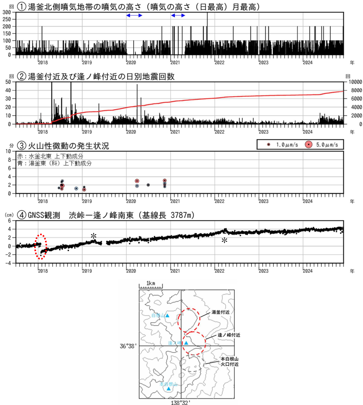
図3 草津白根山（白根山（湯釜付近）） 火山活動経過図（2017年7月1日～2024年11月30日）
