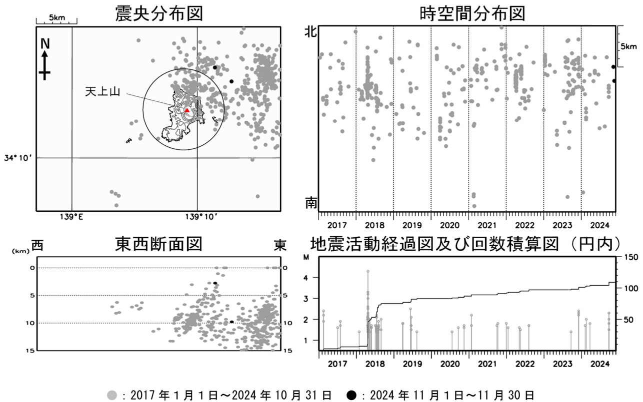
図3 神津島 広域地震観測網による山体・周辺の地震活動（2017年1月1日～2024年11月30日）
