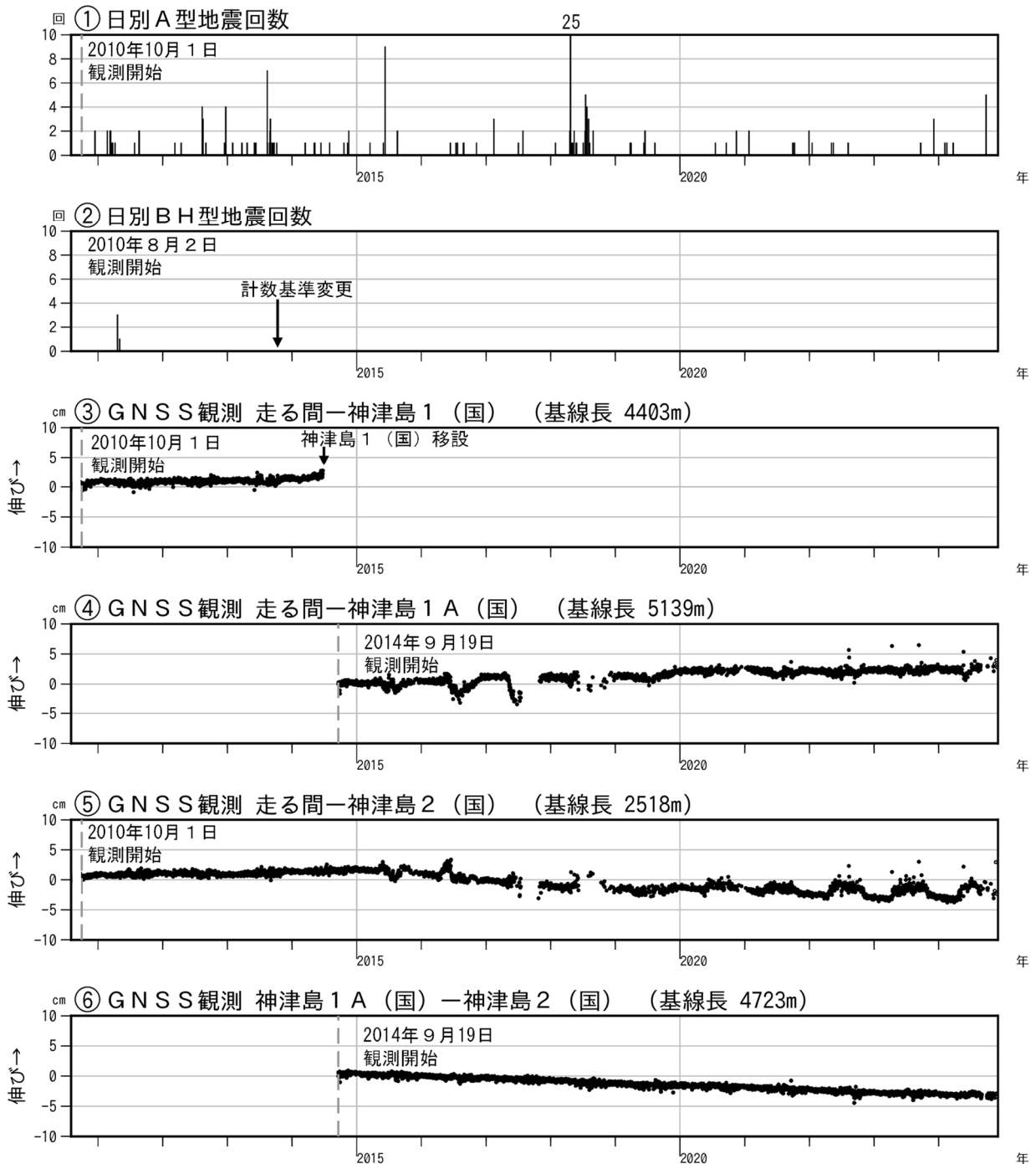
図2 神津島 火山活動経過図(2010年8月2日～2024年11月30日)
