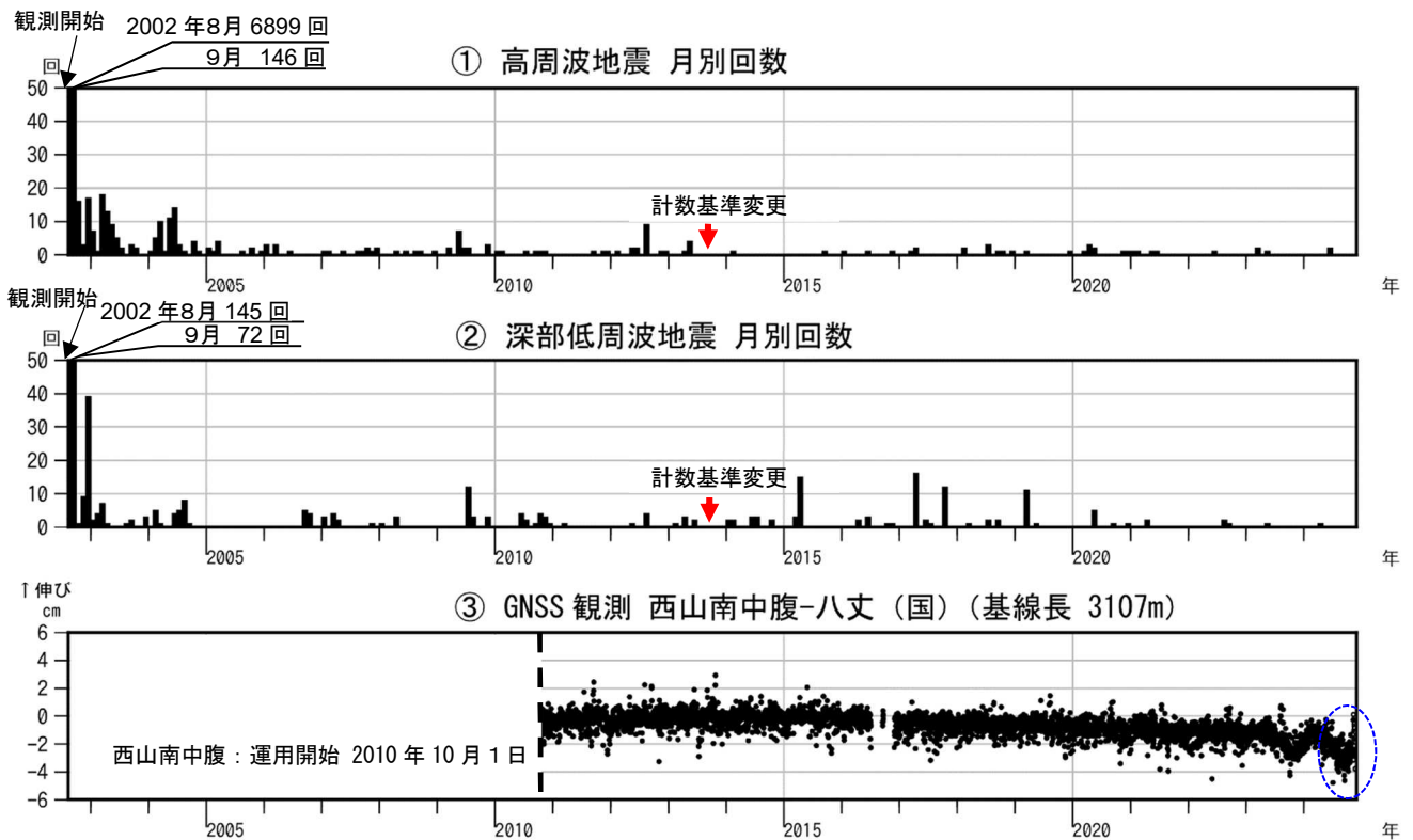
図2 八丈島 火山活動経過図（2002年8月13日～2024年11月30日）
