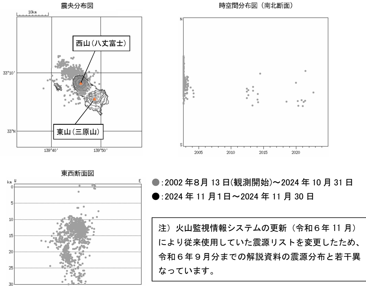
図3 八丈島 震源分布図（2002年8月13日～2024年11月30日）
