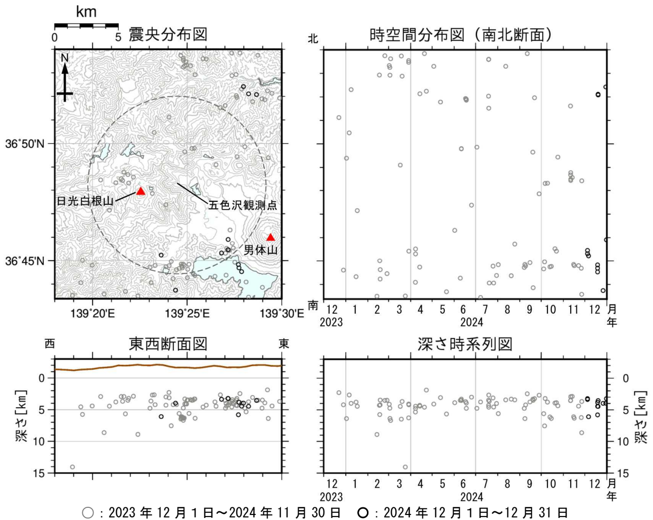
図3 日光白根山 広域地震観測網による山体周辺の地震活動 (2023 年 12 月 1 日～2024 年 12 月 31 日)
