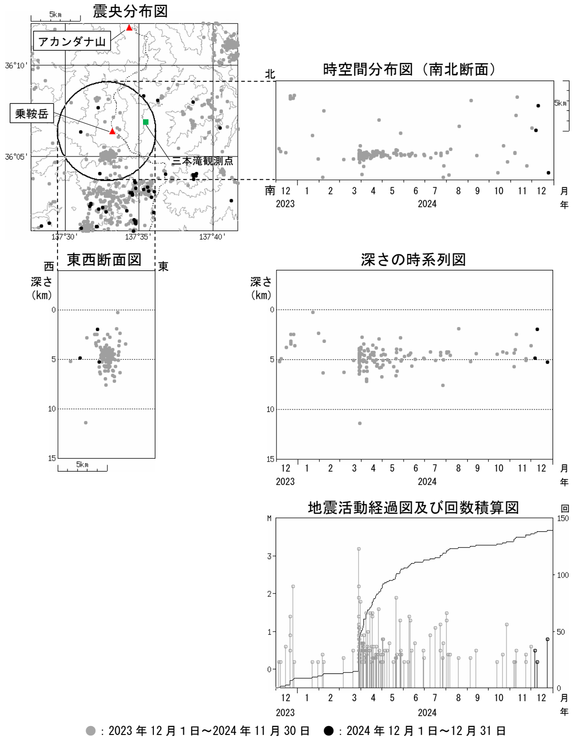
図3 乗鞍岳 広域地震観測網による山体・周辺の地震活動(2023年12月1日～2024年12月31日) M(マグニチュード)は地震の規模を表し、M0.2以上の地震を表示しています。 広域地震観測網により震源決定したもので、深さは全て海面以下として決定しています。なお、2020年9月以降については、地震観測点の標高を考慮する等、震源決定の手法を変更しております。図中の震源要素は一部暫定値が含まれており、後日変更することがあります。 東西断面図、時空間分布図、深さの時系列図、地震活動経過図及び回数積算図には、乗鞍岳付近(震央分布図中の黒線円の範囲)の地震を示しています。 ・3月29日の乗鞍岳の南2km付近を震源とする地震の発生以降、地震回数が増加していましたが、6月以降はこの地震発生以前の地震回数と同程度となっています。
