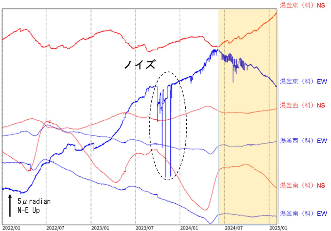
図5 草津白根山（白根山（湯釜付近）） 傾斜変動（2022年1月1日～2025年1月31日） （科）：東京科学大学
