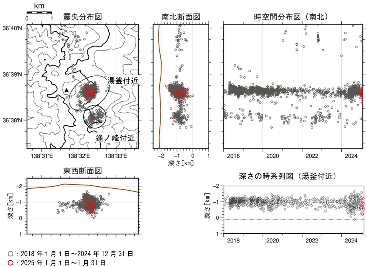
図4 草津白根山 震源分布図（2018 年 1 月 1 日～2025 年 1 月 31 日）
