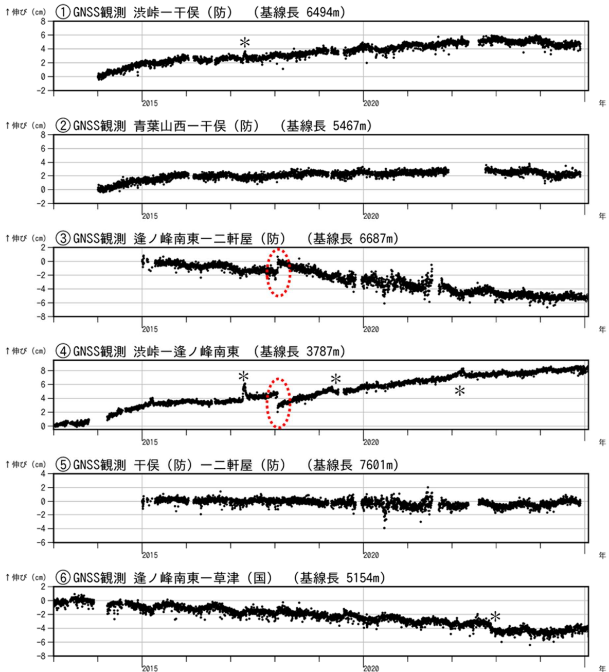
図6 草津白根山 GNSS 連続観測の結果（2013年1月1日～2025年1月31日）
