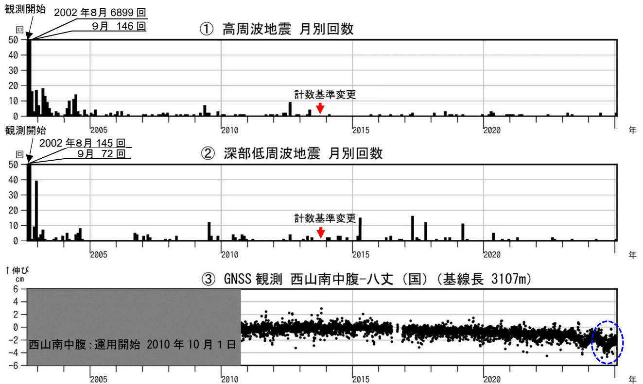
図2 八丈島 火山活動経過図（2002年8月13日～2025年1月31日）
