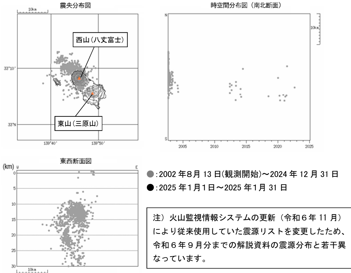
図3 八丈島 震源分布図（2002年8月13日～2025年1月31日）
