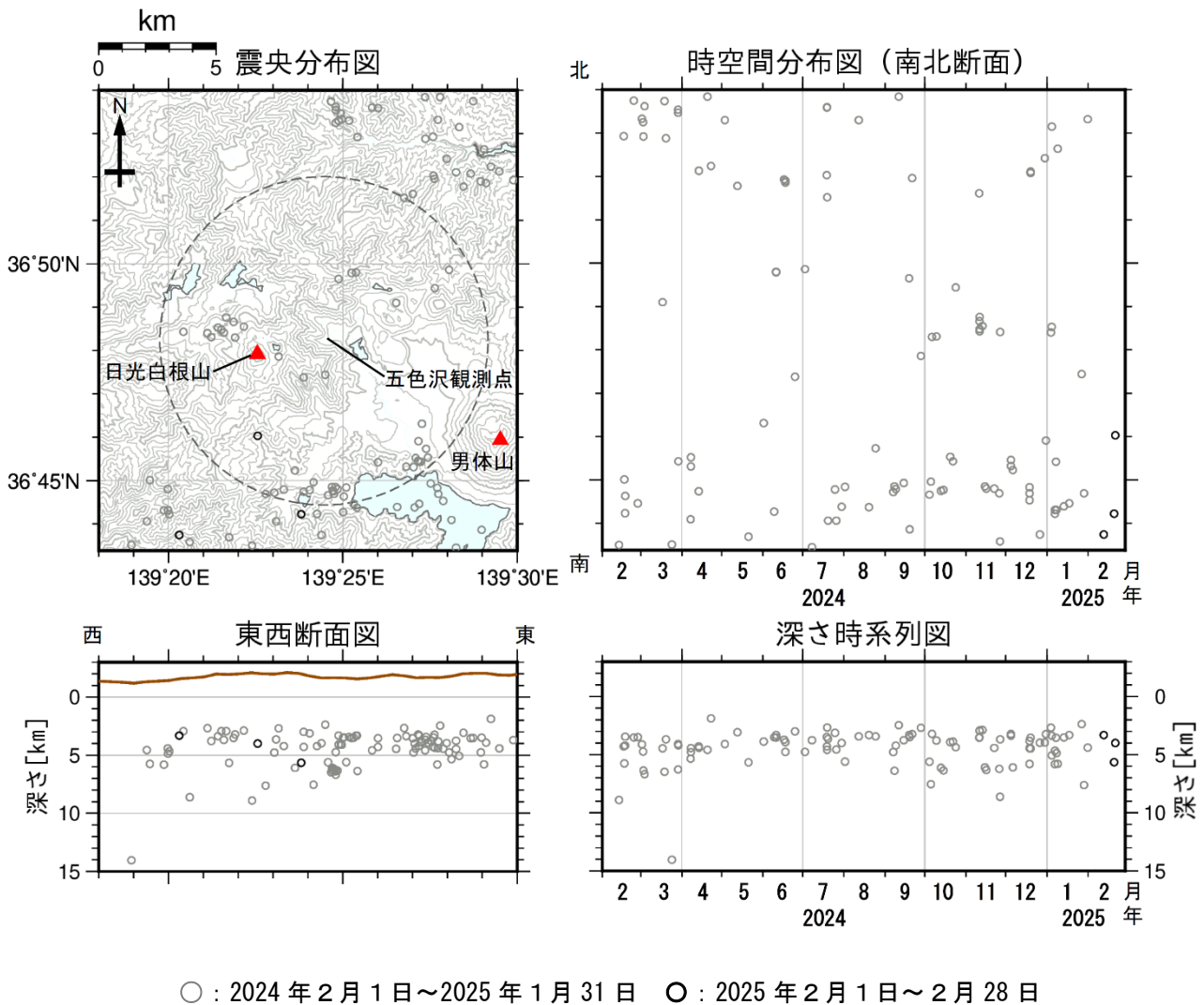
図3 日光白根山 広域地震観測網による山体周辺の地震活動 (2024 年 2 月 1 日～2025 年 2 月 28 日)
