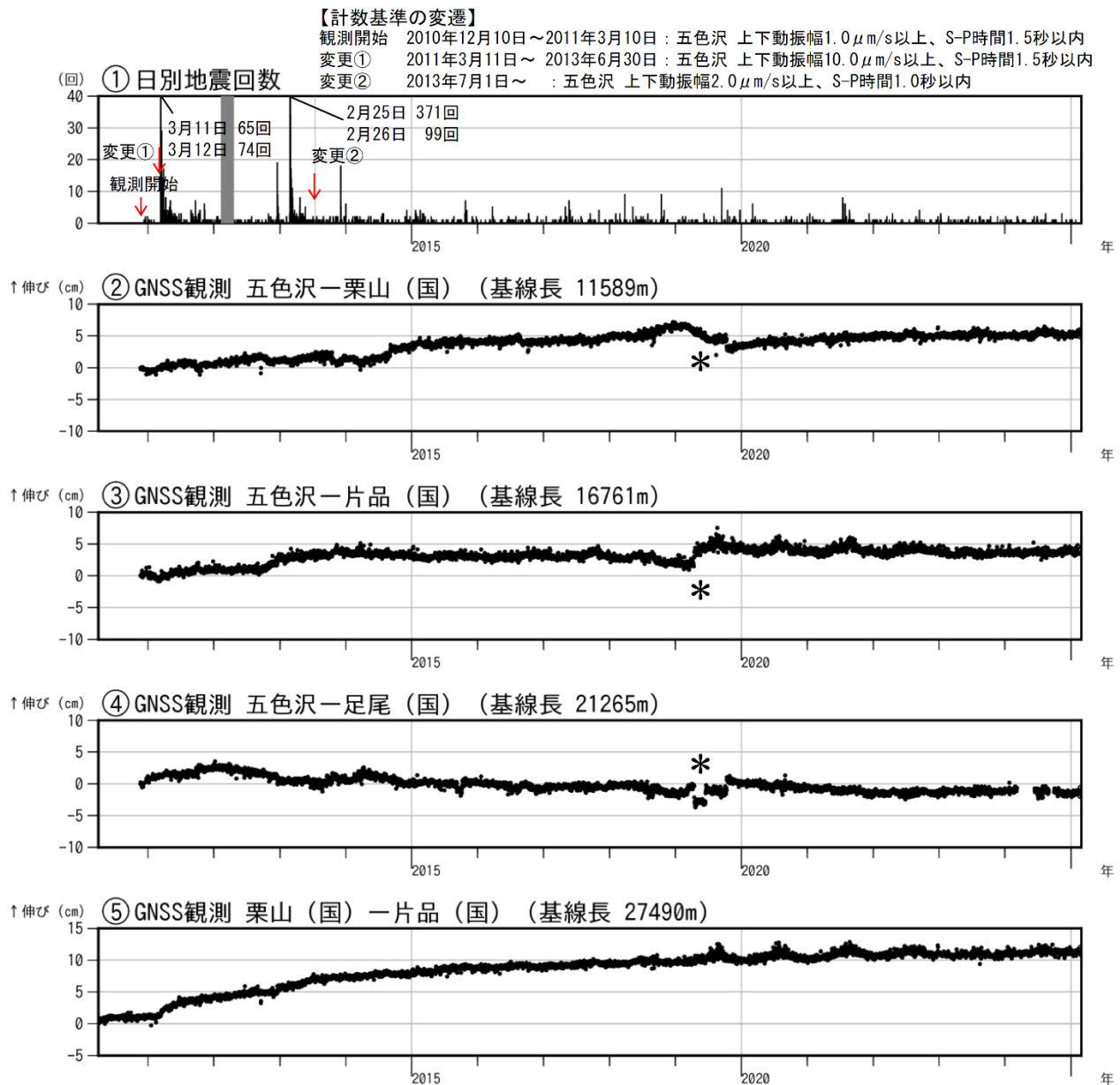
図2 日光白根山 火山活動経過図（2010年4月1日～2025年2月28日）
