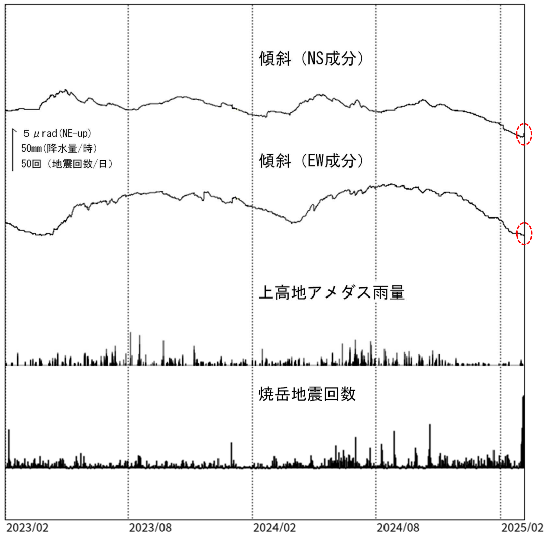
図8－1 焼岳 南峰南東観測点における傾斜データ（2023年2月1日～2025年3月8日）
