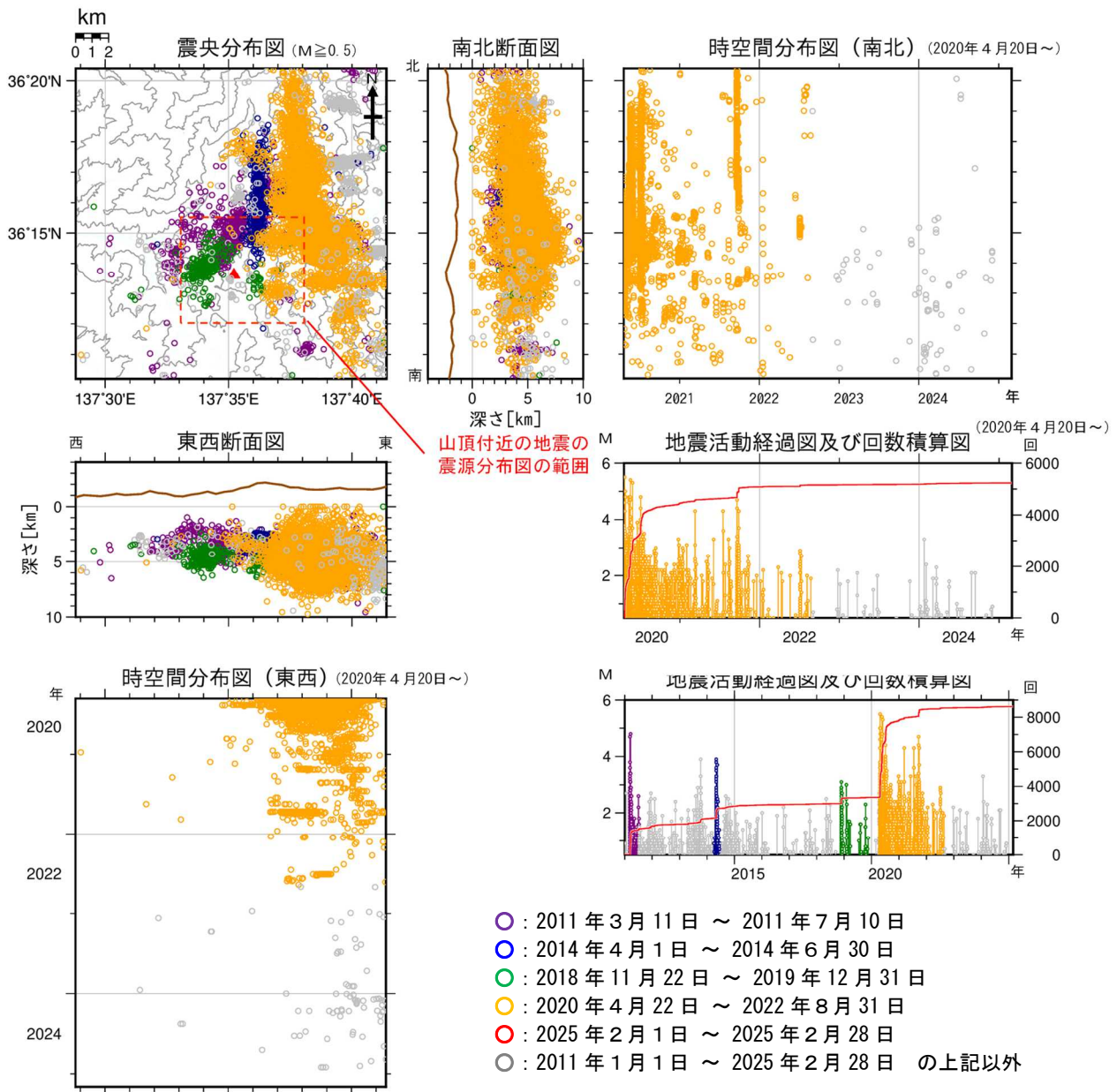
図9 焼岳 広域地震観測網による山体及び周辺の地震活動(2011年1月1日～2025年2月28日)
