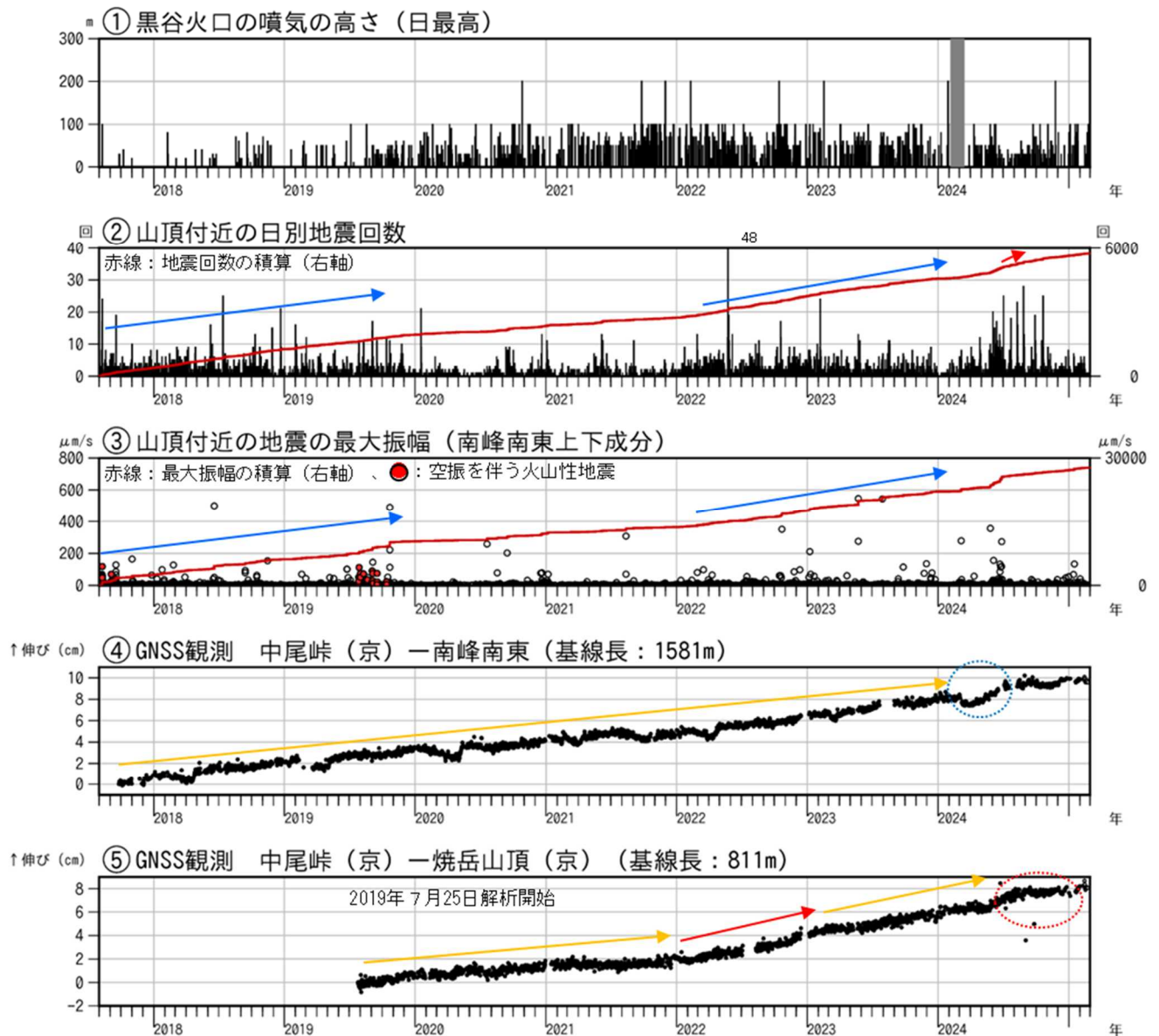
図1—1 焼岳 火山活動経過図（2017年8月1日～2025年2月28日）
