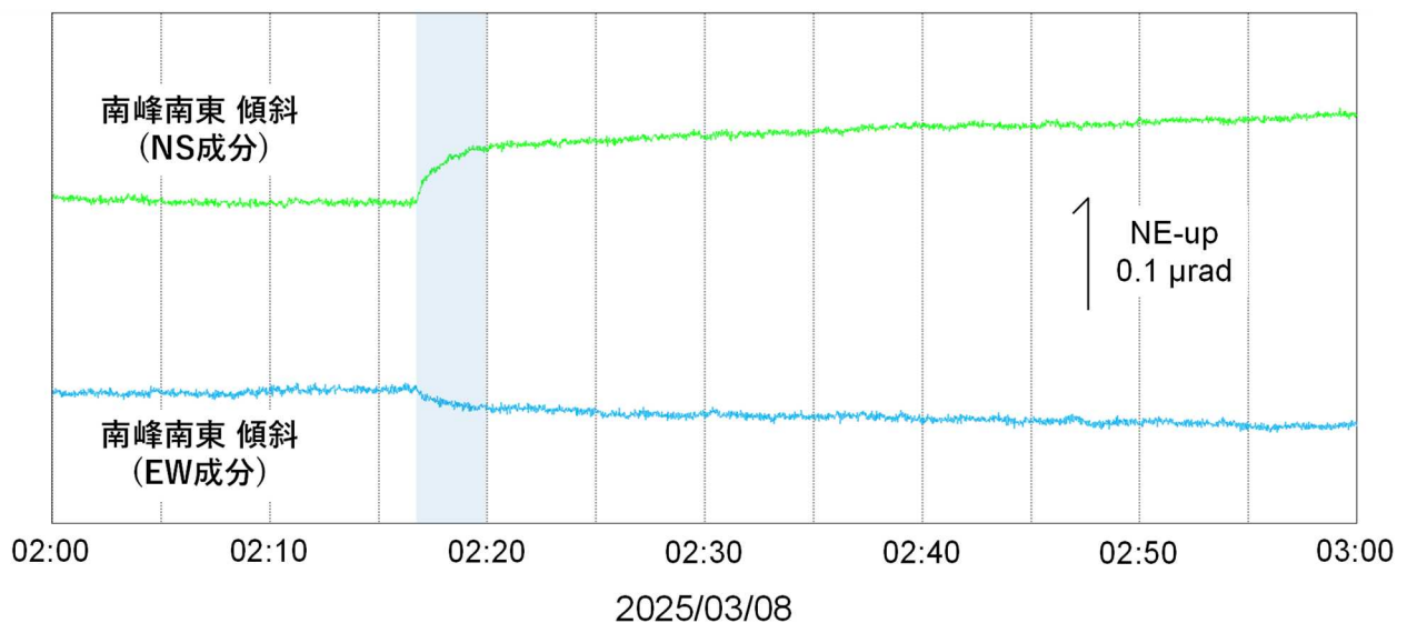
図8－3 焼岳 3月8日（期間外）に観測された傾斜変動（02時00分～03時00分）
