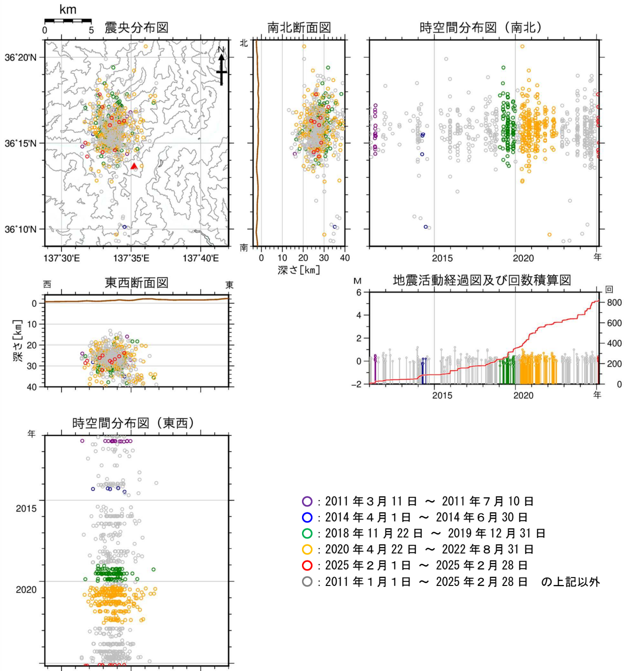
図10 焼岳 広域地震観測網による深部低周波地震の震源分布図（2011年1月1日～2025年2月28日）
