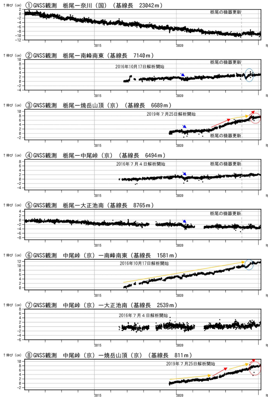
図6 焼岳 GNSS 連続観測による基線長変化（2010年10月1日～2025年2月28日）
