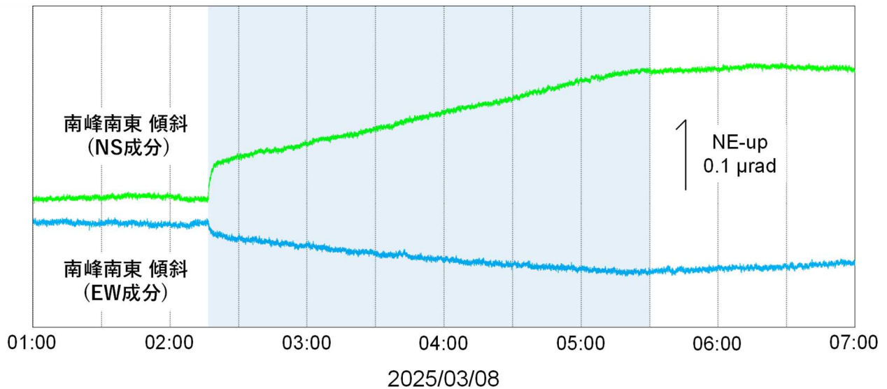
図8－2 焼岳 3月8日（期間外）に観測された傾斜変動（01時00分～07時00分）
