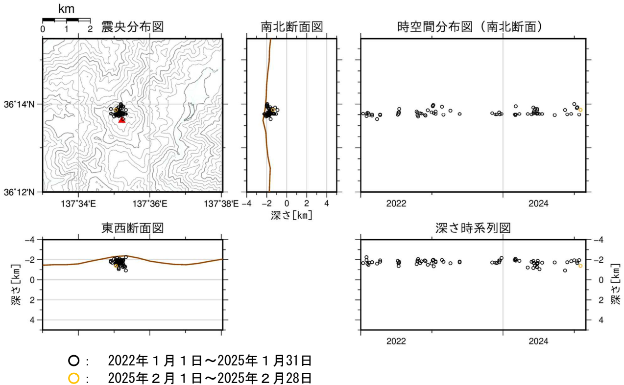
図2 焼岳 山頂付近の地震の震源分布図（2022年1月1日～2025年2月28日）
