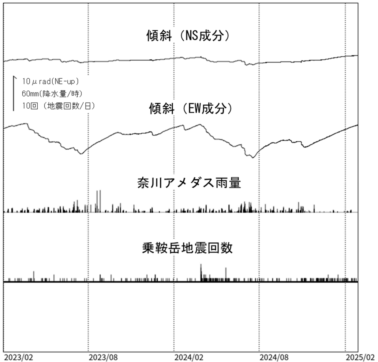
図4 乗鞍岳 三本滝観測点における傾斜データ（2023年2月1日～2025年2月28日） ・傾斜計による観測では、火山活動によるとみられる変動は認められません。
