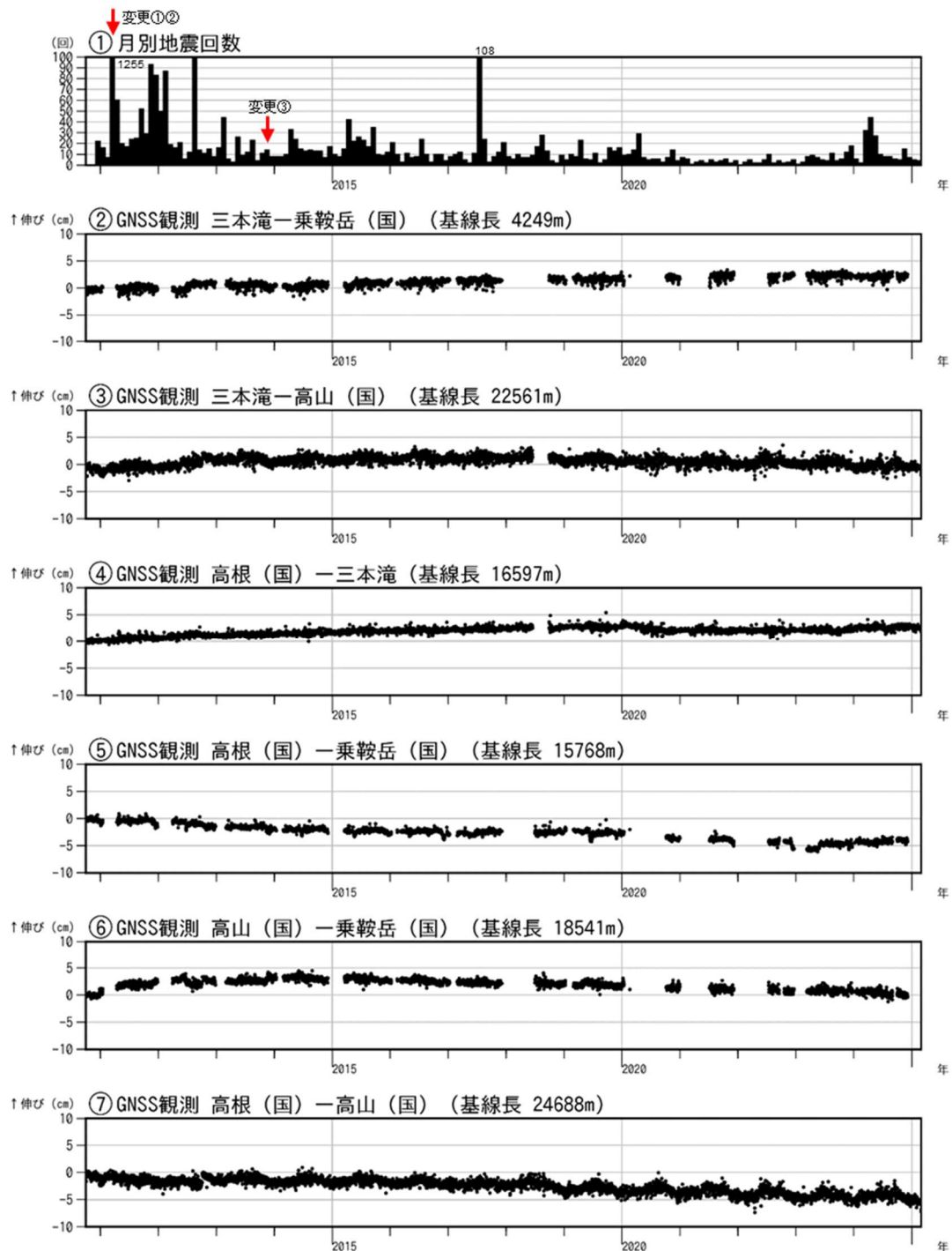
図2 乗鞍岳 火山活動経過図（2010年10月1日～2025年2月28日）
