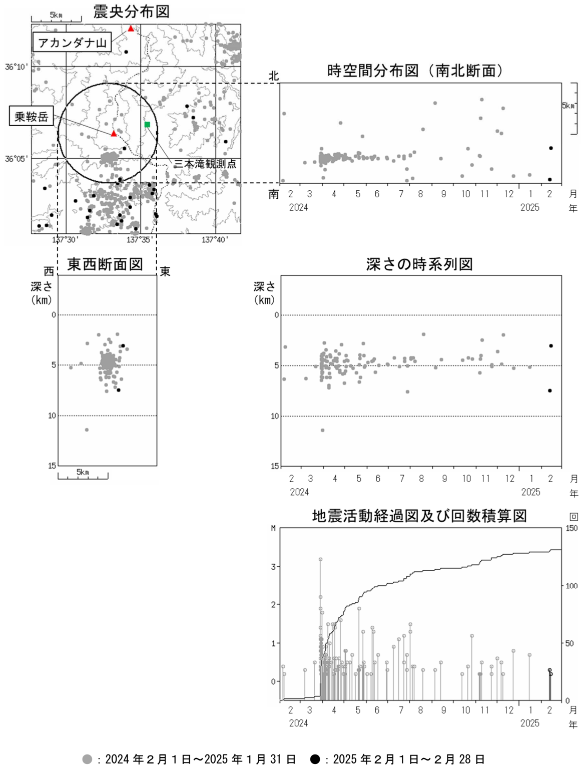
図3 乗鞍岳 広域地震観測網による山体・周辺の地震活動(2024年2月1日～2025年2月28日)
