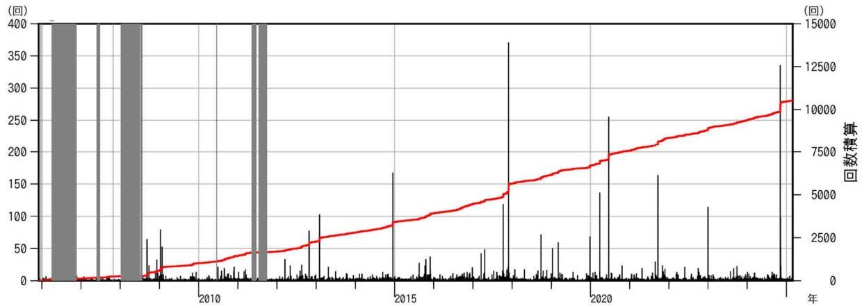
図3 白山 日別地震回数と積算回数（2005年12月1日～2025年2月28日） 図の灰色部分は機器障害による欠測期間。
