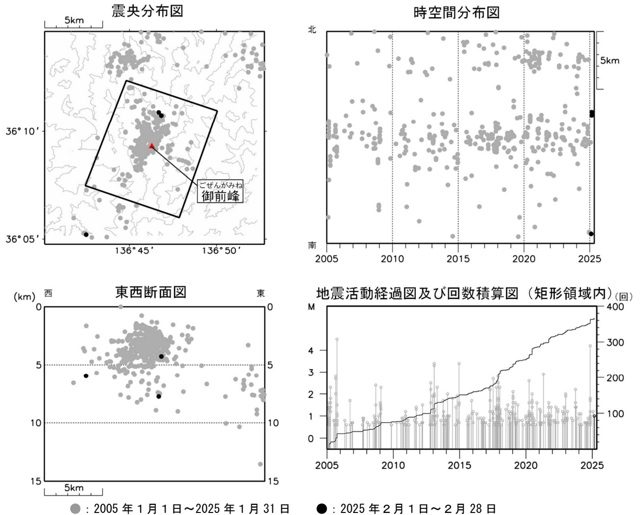
図4 白山 広域地震観測網による山体・周辺の地震活動（2005年1月1日～2025年2月28日） 広域地震観測網により震源決定したもので、深さは全て海面以下として決定しています。なお、2020年9月以降については、地震観測点の標高を考慮する等、震源決定の手法を変更しております。 M（マグニチュード）は地震の規模を表します。M0.6以上の地震を表示しています。 図中の震源要素は一部暫定値を含んでおり、後日変更することがあります。 ・今期間、白山付近の地震活動は低調に経過しました。
