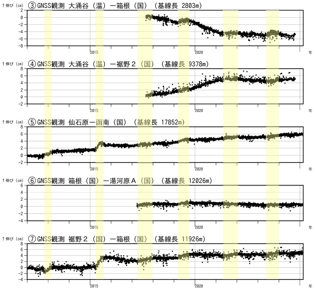
図3-2 箱根山 GNSS連続観測による 基線長変化及び観測点配置図 (2012年1月1日～2025年2月28日)
