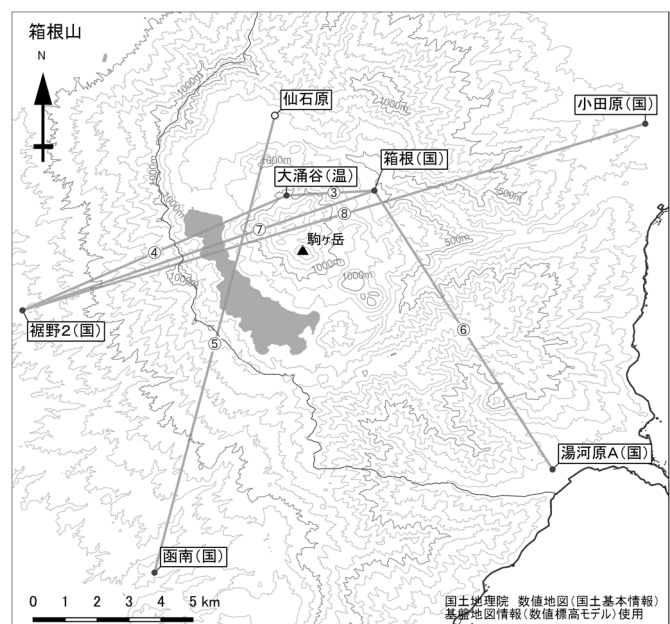
図3-2 箱根山 GNSS連続観測による 基線長変化及び観測点配置図 (2012年1月1日～2025年2月28日)
