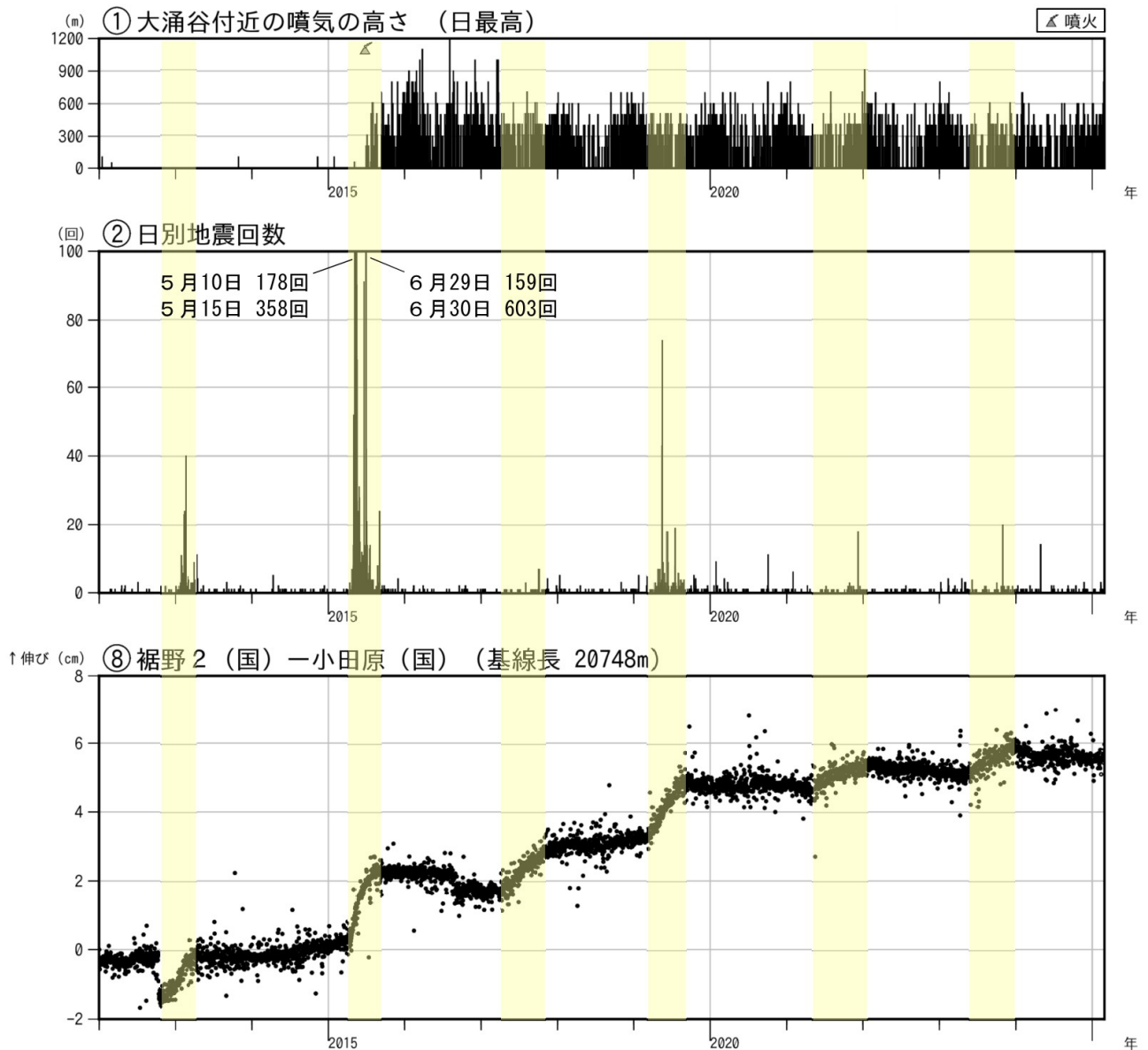
図3-1 箱根山 火山活動経過図（2012年1月1日～2025年2月28日）
