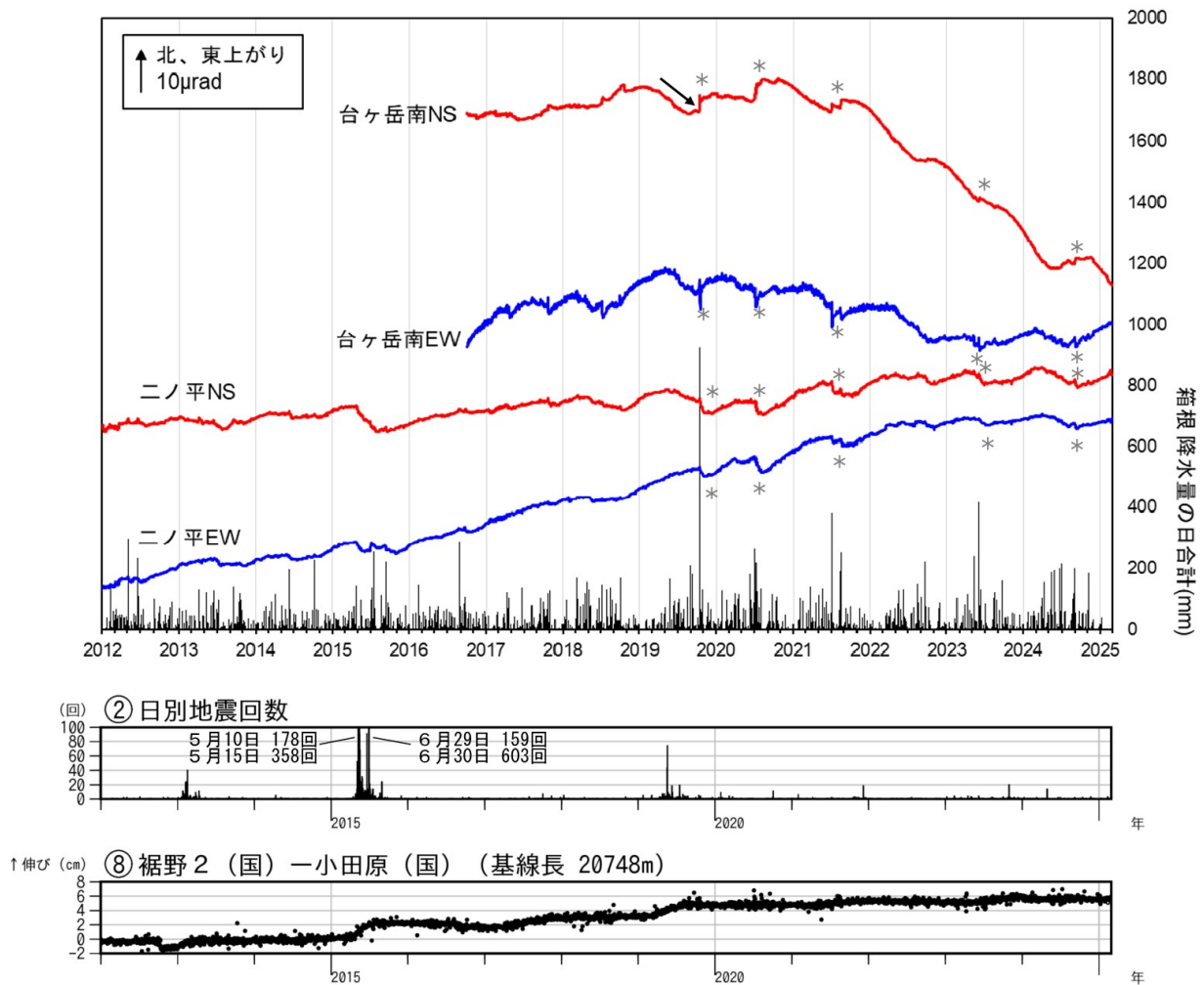
図5 箱根山 傾斜観測及び地震回数・GNSS観測（2012年1月1日～2025年2月28日）
