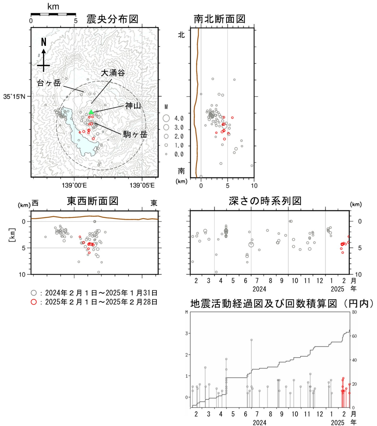
図4 箱根山 広域地震観測網による山体周辺の震源分布図（2024年2月1日～2025年2月28日）
