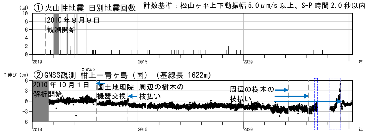
図2 青ヶ島 火山活動経過図 (2010年8月9日～2025年2月28日)
