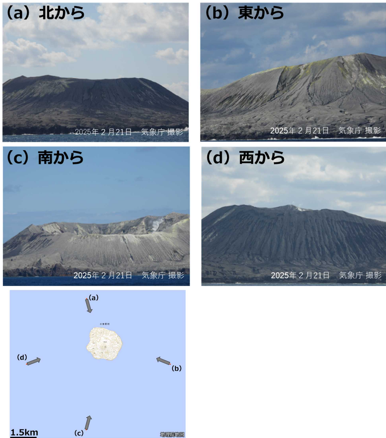
図3 西之島 海上からの観測による西之島の状況（21日 海洋気象観測船「啓風丸」観測）
