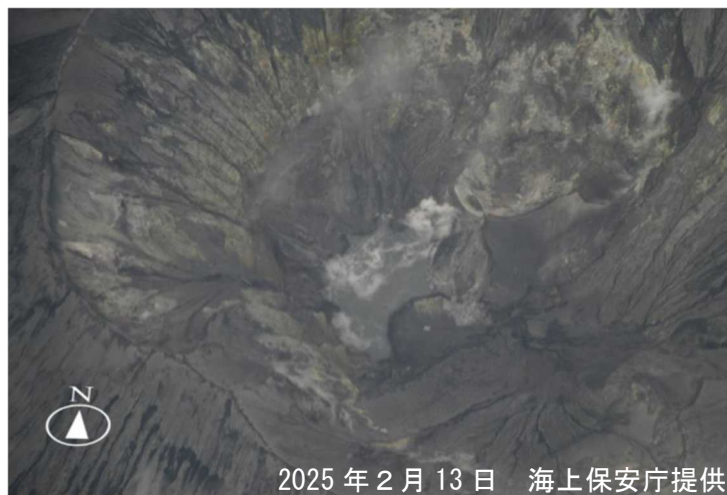
図2 西之島 上空からの観測による西之島の状況（2月13日 海上保安庁による観測）
