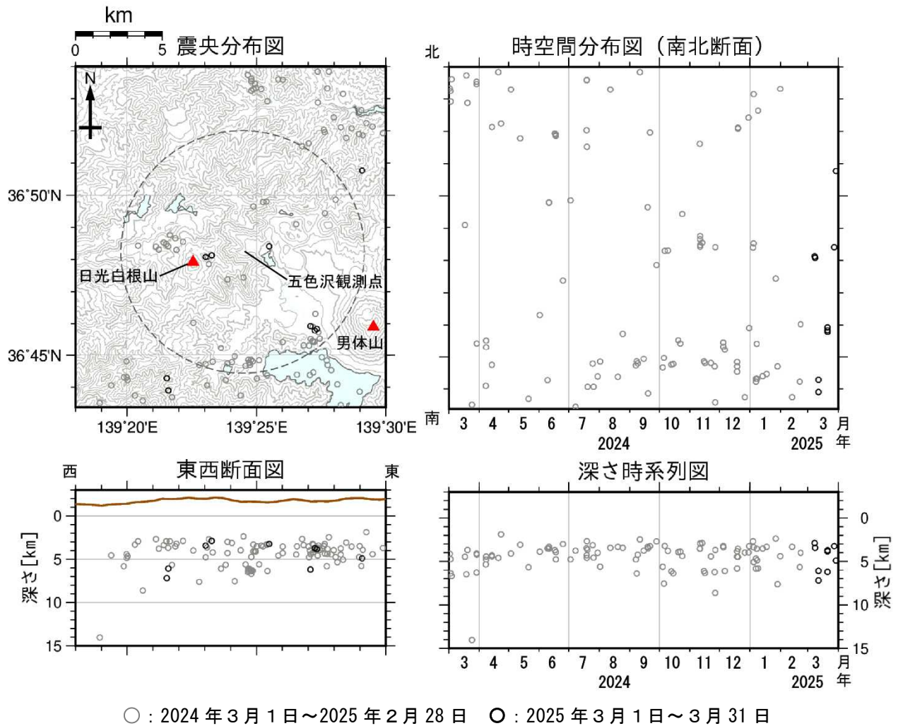
図3 日光白根山 広域地震観測網による山体周辺の地震活動 (2024 年 3 月 1 日～2025 年 3 月 31 日)
