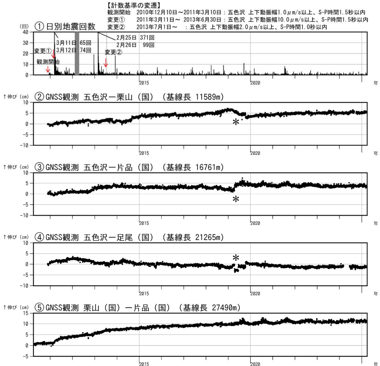
図2 日光白根山 火山活動経過図（2010年4月1日～2025年3月31日）
