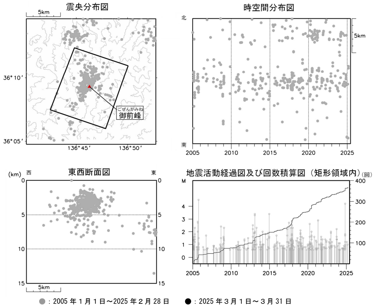
図4 白山 広域地震観測網による山体・周辺の地震活動（2005年1月1日～2025年3月31日）
