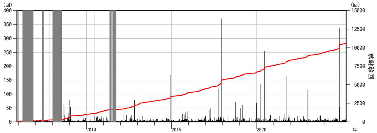
図3 白山 日別地震回数と積算回数（2005年12月1日～2025年3月31日）
