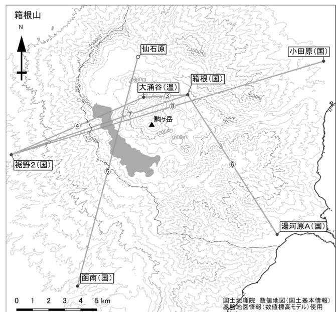
図3-2 箱根山 GNSS連続観測による 基線長変化及び観測点配置図 (2012年1月1日～2025年3月31日)
