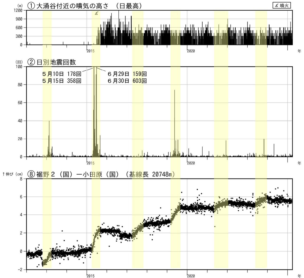
図 3 - 1 箱根山 火山活動経過図（2012 年 1 月 1 日～2025 年 3 月 31 日）
