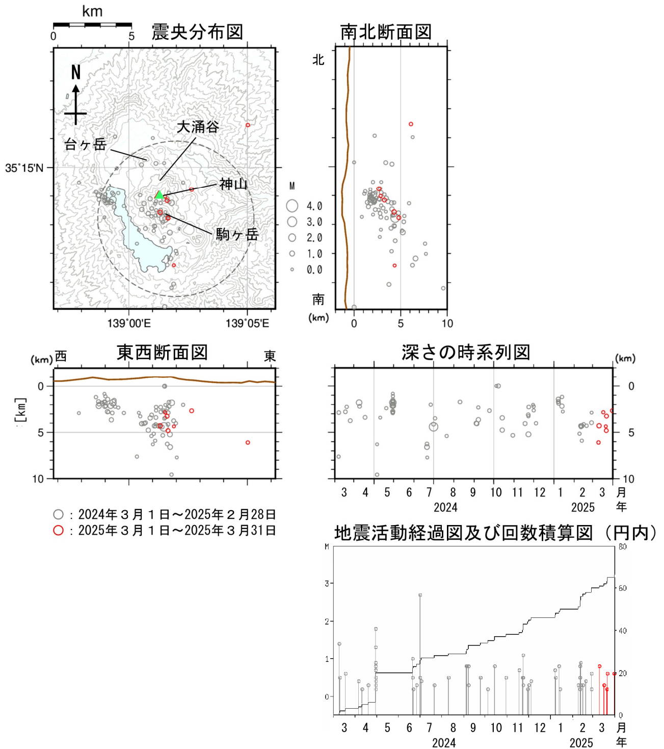
図4 箱根山 広域地震観測網による山体周辺の震源分布図（2024年3月1日～2025年3月31日）
