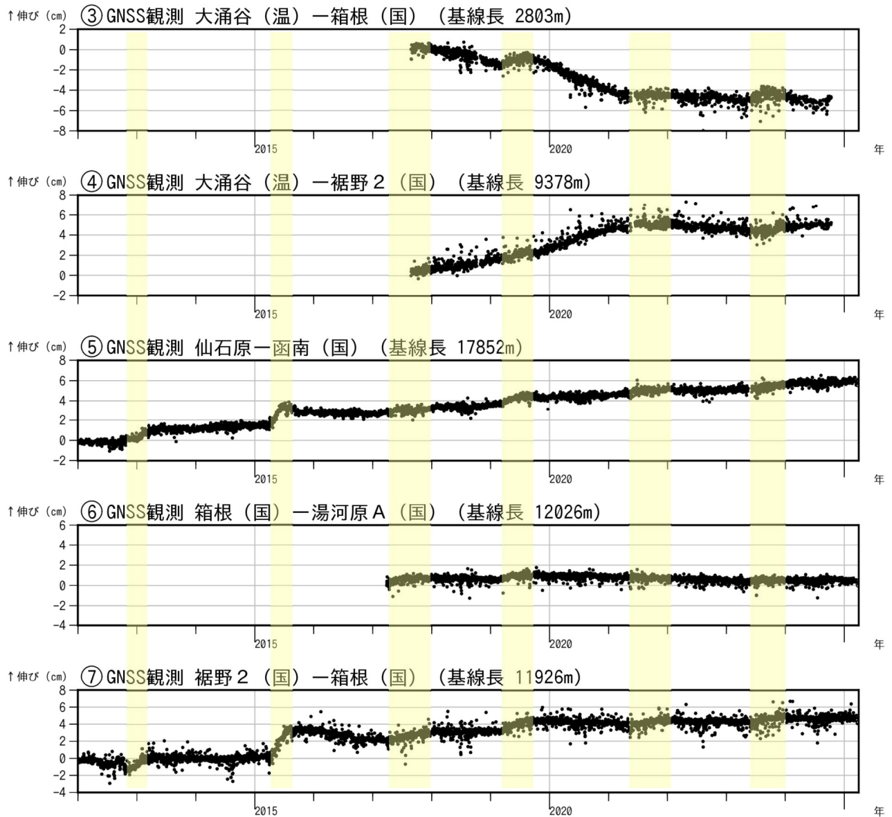
図3-2 箱根山 GNSS連続観測による 基線長変化及び観測点配置図 (2012年1月1日～2025年3月31日)
