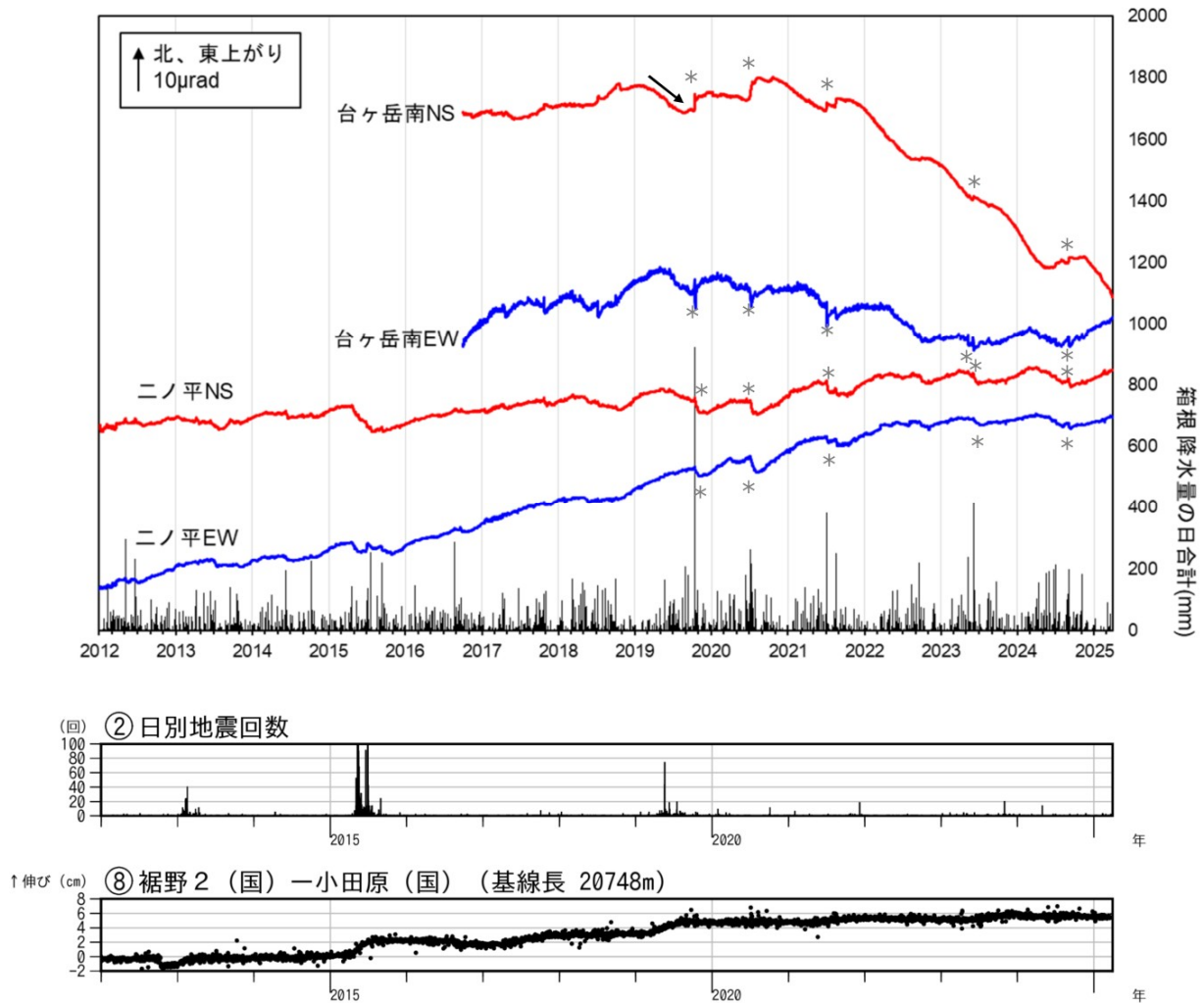
図5 箱根山 傾斜観測及び地震回数・GNSS観測（2012年1月1日～2025年3月31日）
