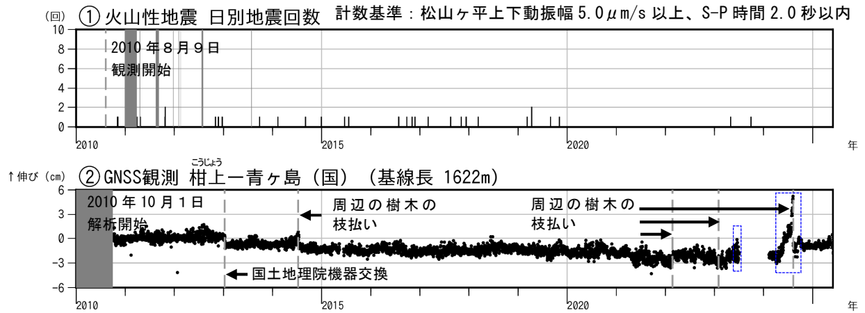
図2 青ヶ島 火山活動経過図（2010年8月9日～2025年5月31日）
